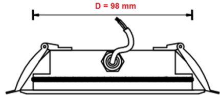
Montage in der Decke
