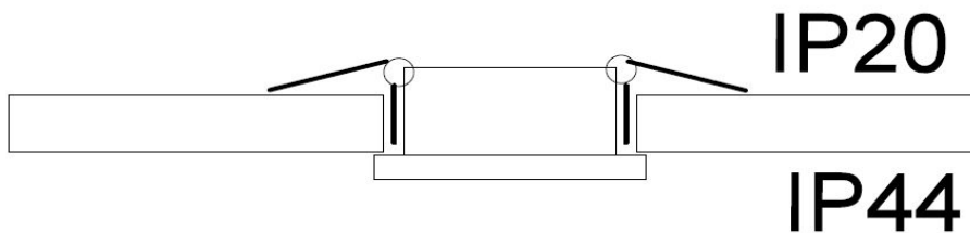
Abb.: 3 Einbau in geschlossene Decken
