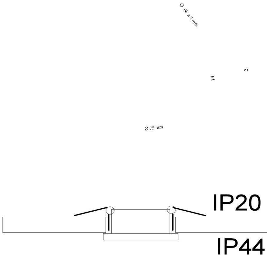
Abb.: 2 Einbau in geschlossene Decken
