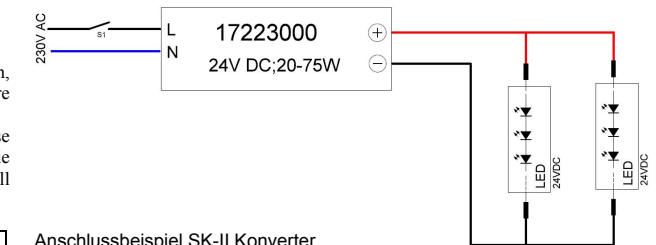
Anschlussbeispiel SK-II Konverter
