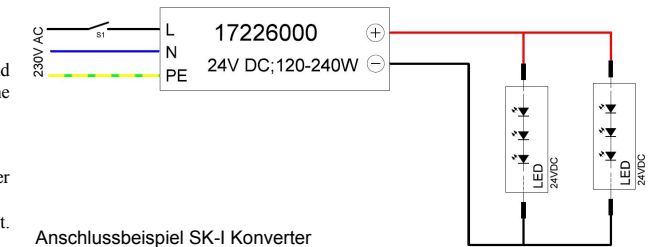
Anschlussbeispiel SK-I Konverter
